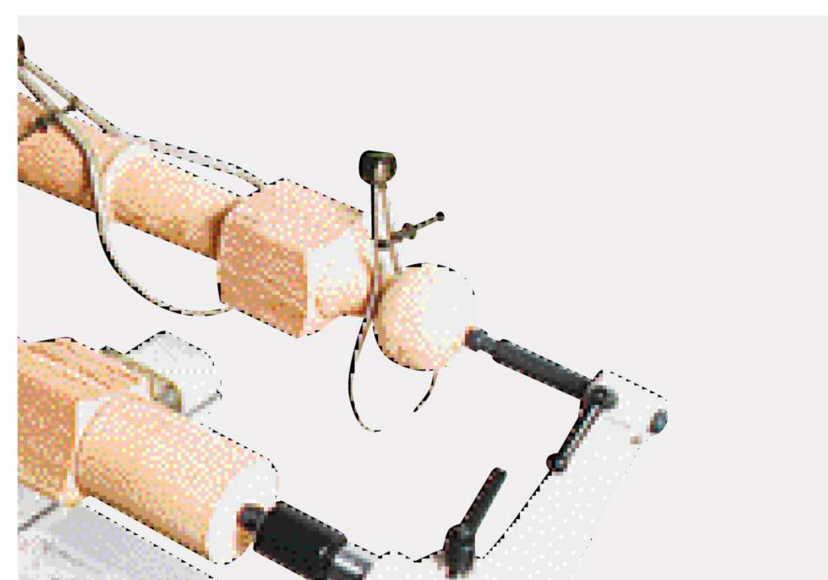
Zentrierspitzen ermöglichen das Aufspannen eines Musterwerkstückes
